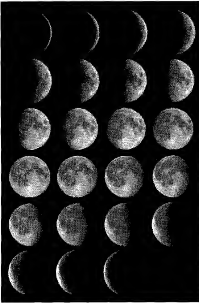
صورة توضح التدرج في زيادة الجزء المنير من سطح القمر مع الزمن في كل شهر قمري ثم تناقصه إلى المحاق .
